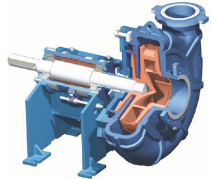
Pompe Metso série Orion, coupes de pompes HM (revêtement métallique) et HR (revêtement caoutchouc) pompes à boue horizontales extra robuste.
