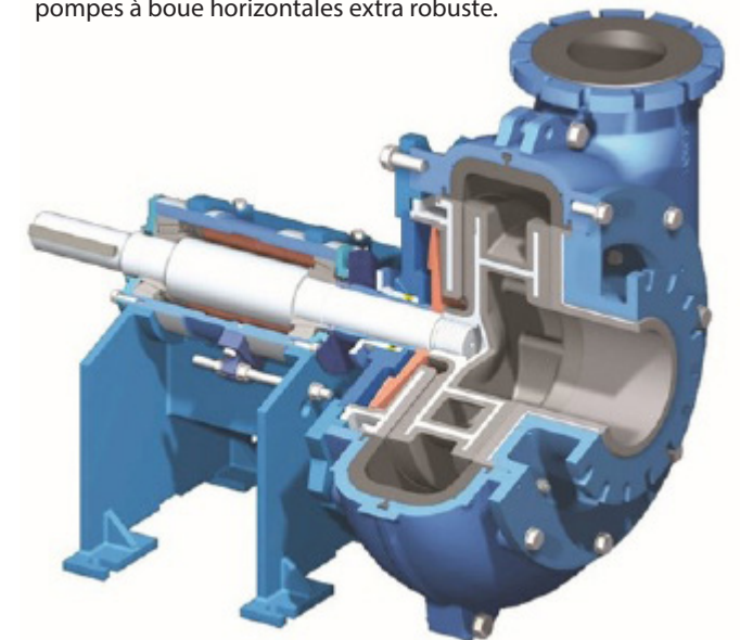
Pompe Metso série Orion, coupes de pompes HM (revêtement métallique) et HR (revêtement caoutchouc) pompes à boue horizontales extra robuste.
