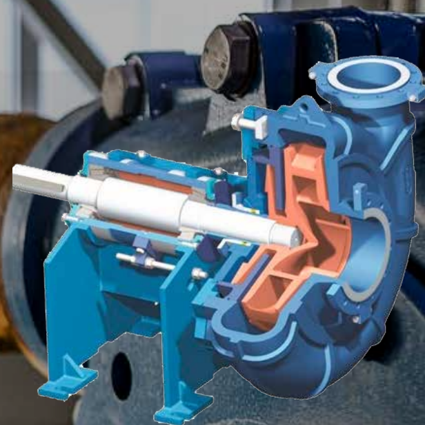
Bombas Metso de la serie Orion, sección de bombas HM (revestimiento de metal) y HR (revestimiento de goma), bombas de lodo horizontales extra resistentes.
